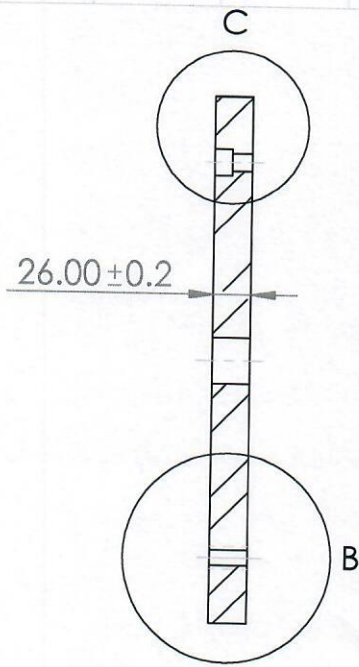
SECTION A-A SCALE 1 : 5
