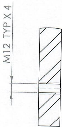
SECTION A-A SCALE 1 : 5
