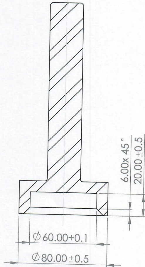
SECTION A-A
