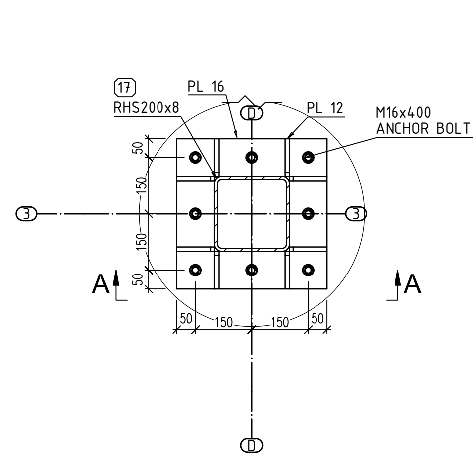
DETAIL A 002-Anchor Scale: 1:10
